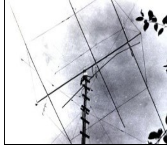
Перша в Умані обертова антена QUAD – Олександра Мельника UB5CAT – 2EL на 14 МГц і 3EL на 21-28 МГц (1974 р.).
