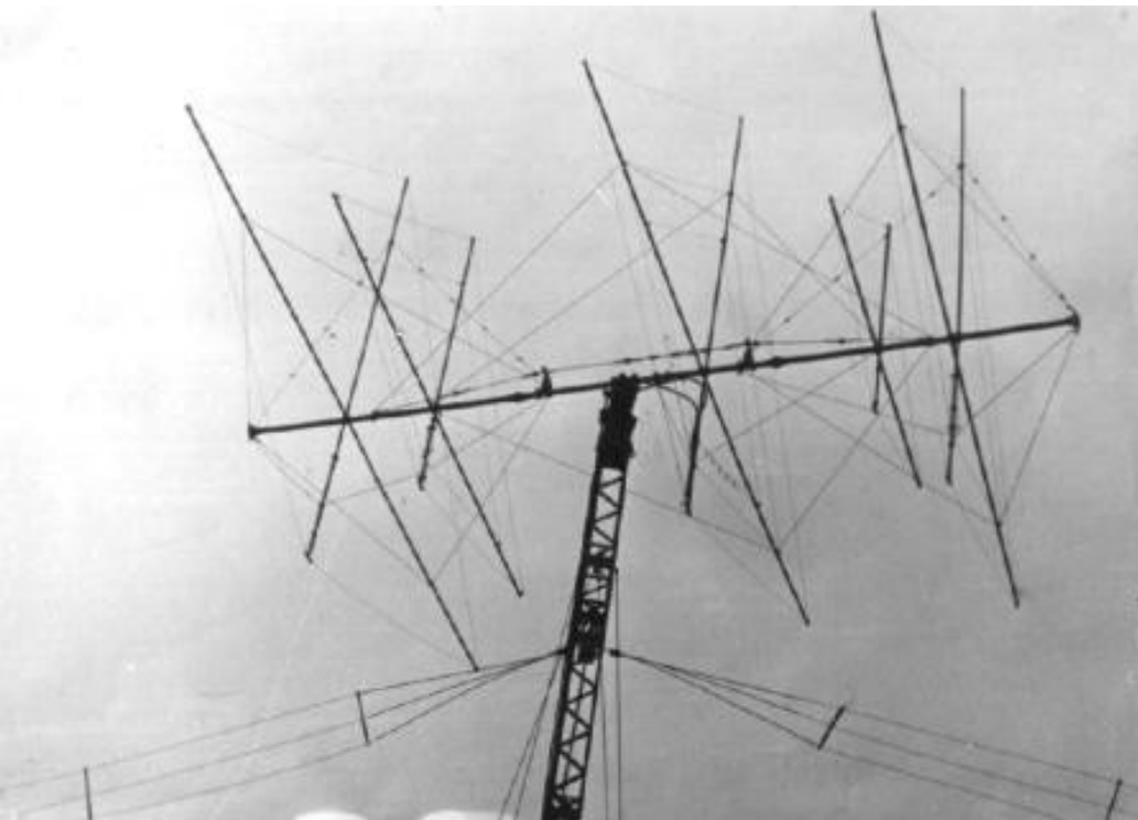
За проектом Олександра Мельника група уманських короткохвильовиків створила антени «Триелементний квадрат» на 14 МГц та чотири-елементний – на 28 та 21 МГц на колективній радіостанції UK5CAP (1980 р.).
